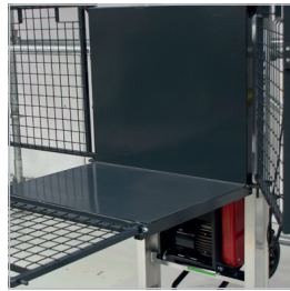
STANDARDNÍ VOZÍK S KLEČÍ 643×800×725 mm
