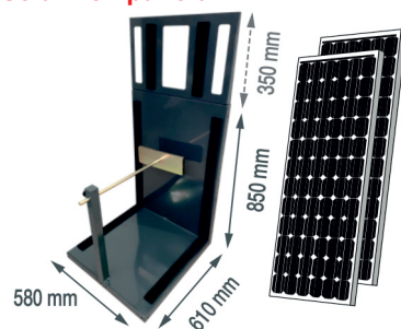
Plošina pro přepravu solárních panelů
